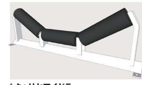
■キャリアアイドラ 株式会社JRC
